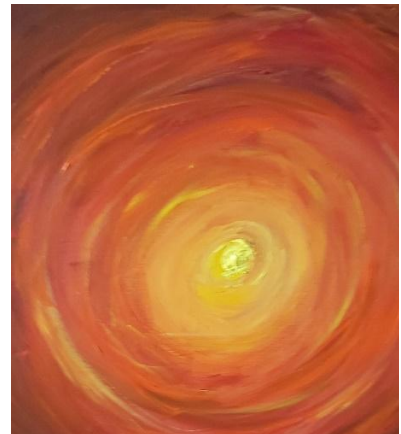
Der erste Spiralnebel bildet sich
